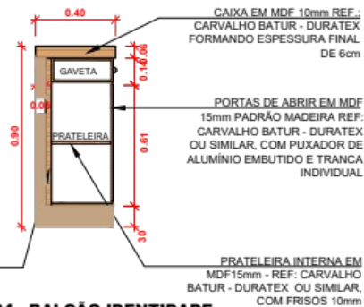
ITEM 04 - BALCÃO IDENTIDADE CORTE Esc 1:25
