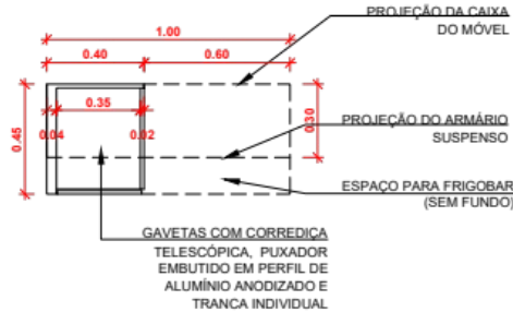
ITEM 06 - ARMÁRIO ALTO SALA ADVOGADAS PLANTA-BAIXA Esc 1:25
