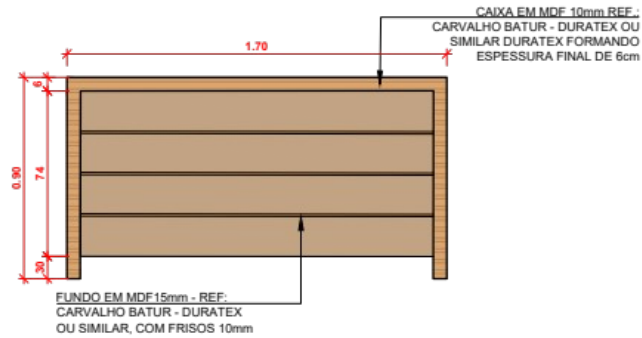
ITEM 04 - BALCÃO IDENTIDADE VISTA FRONTAL Esc 1:25
