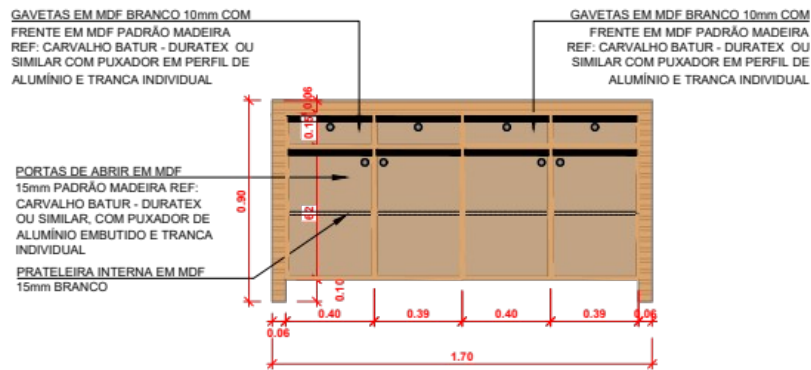
ITEM 04 - BALCÃO IDENTIDADE VISTA POSTERIOR Esc 1:25
