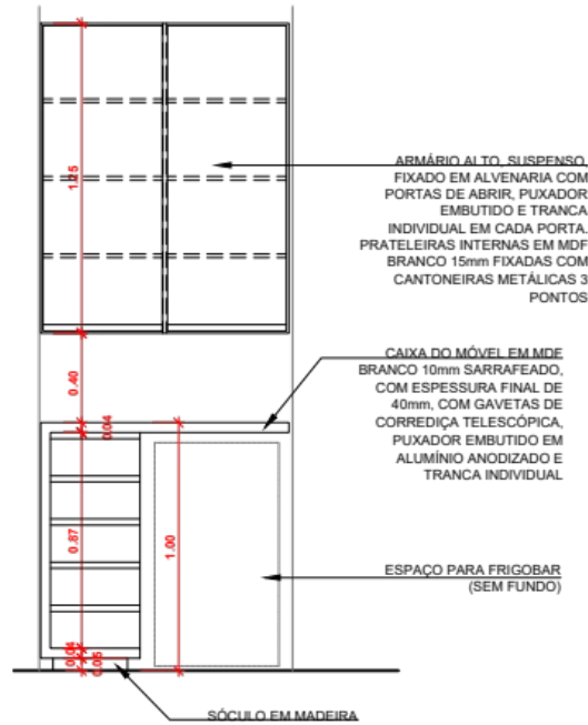
ITEM 06 - ARMÁRIO ALTO SALA ADVOGADAS VISTA FRONTAL Esc 1:25
